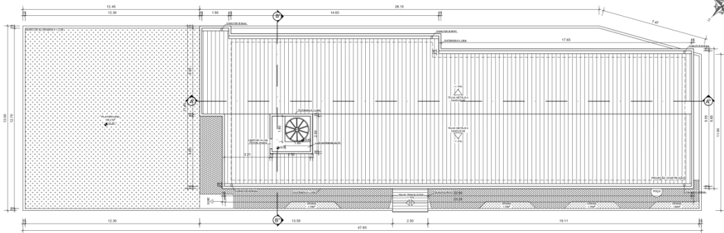
PLANTA DE COBERTURA E IMPLANTAÇÃO ESCALA: 1/1100
