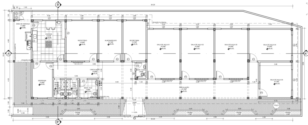
PLANTA PAVIMENTO TÉRREO ESCALA: 1/175
