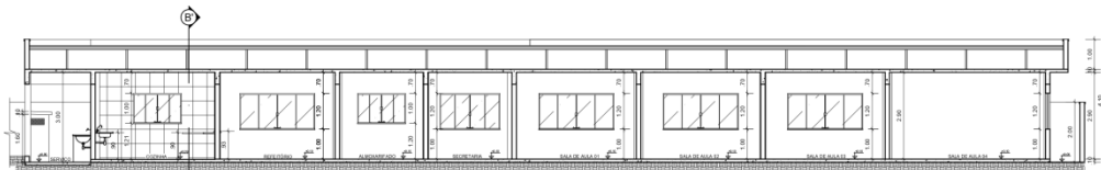
CORTE A-A ESCALA: 1/175
