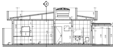
CORTE B-B ESCALA: 1/175
